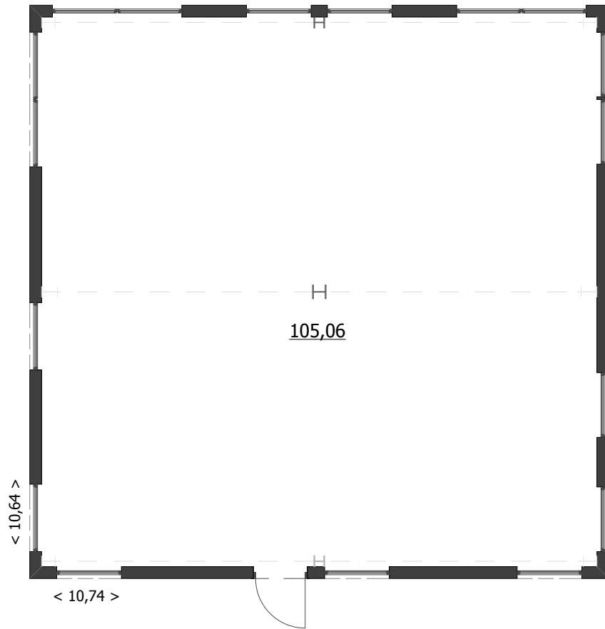
План 1-го этажа на отм. 0,000м (М1:100)
